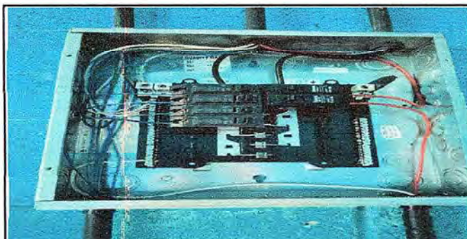
Foto 3: La imagen demuestra las conexiones eléctricas correctas y necesarias en el Ventro Educativo.
